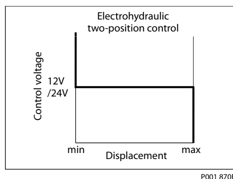
Control operation E1A5, E2A5
